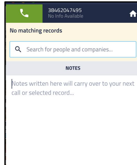
No Match
